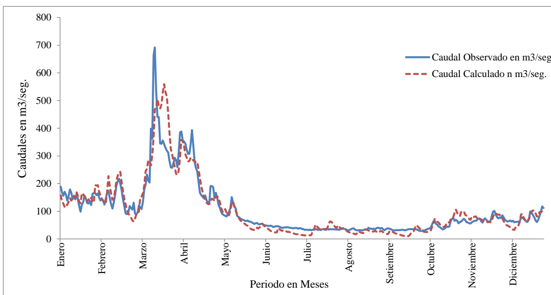
Figura 4.22: Simulación y validación del modelo SRM para el año 2007 en la sub-cuenca Alto Santa – área con glaciares.
