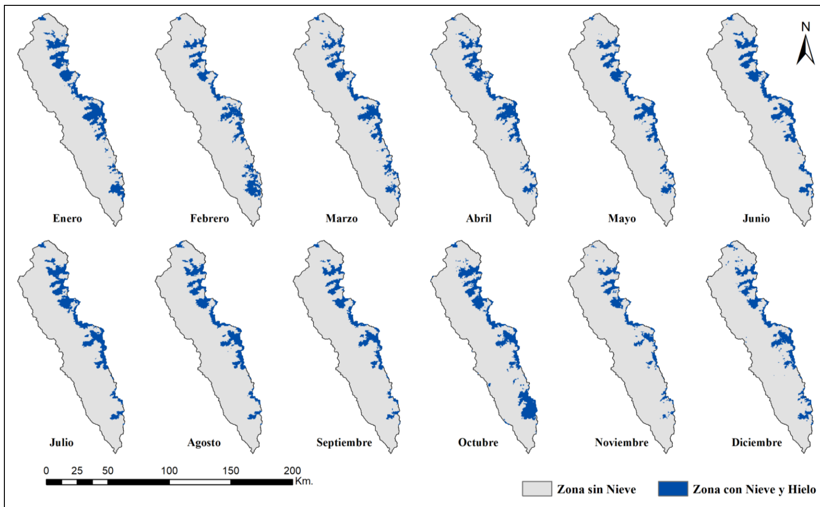
Figura 3.17: Mapas mensuales de cobertura glaciar del año 2017, producto de la imagen de satélite MODIS10A1.
