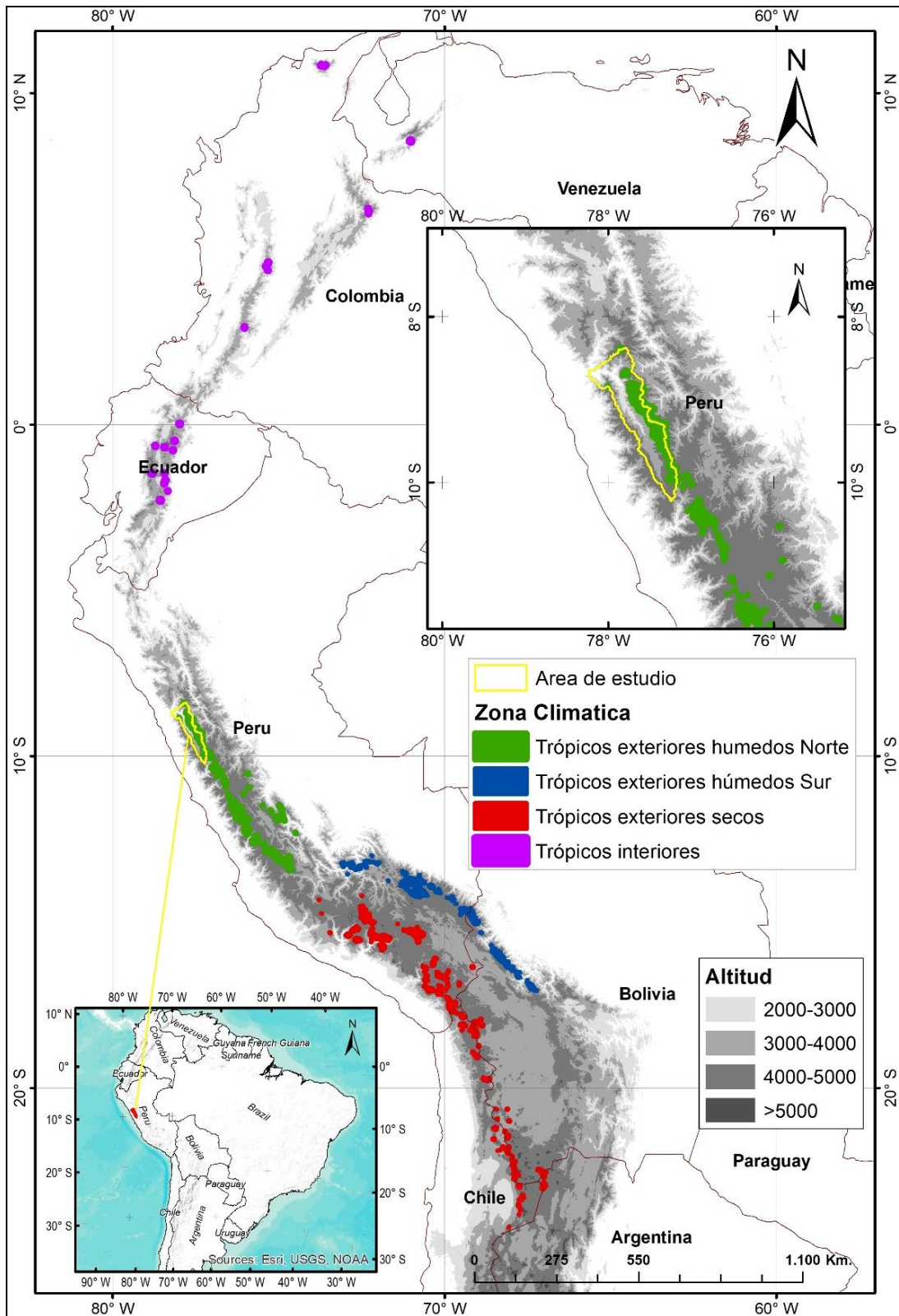
Figura 3.2: Ubicación del área de estudio, sub-cuenca alto Santa, área con glaciares. Fuente: Veettil et al. (2017).
