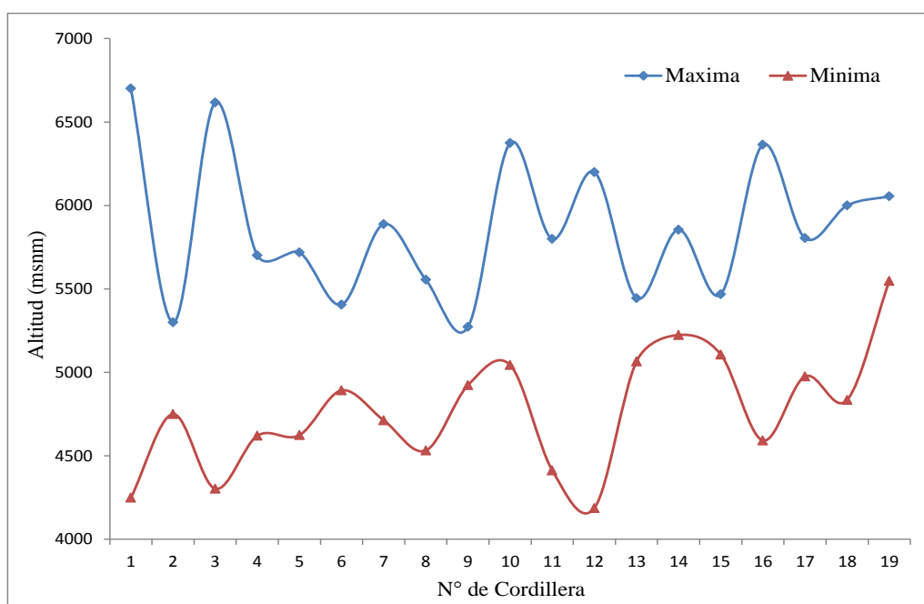
Figura 2.8: Distribución de las altitudes mínimas y máximas de los glaciares, inventario en el año 2014, elaborado con respecto al (Cuadro 2.2).
