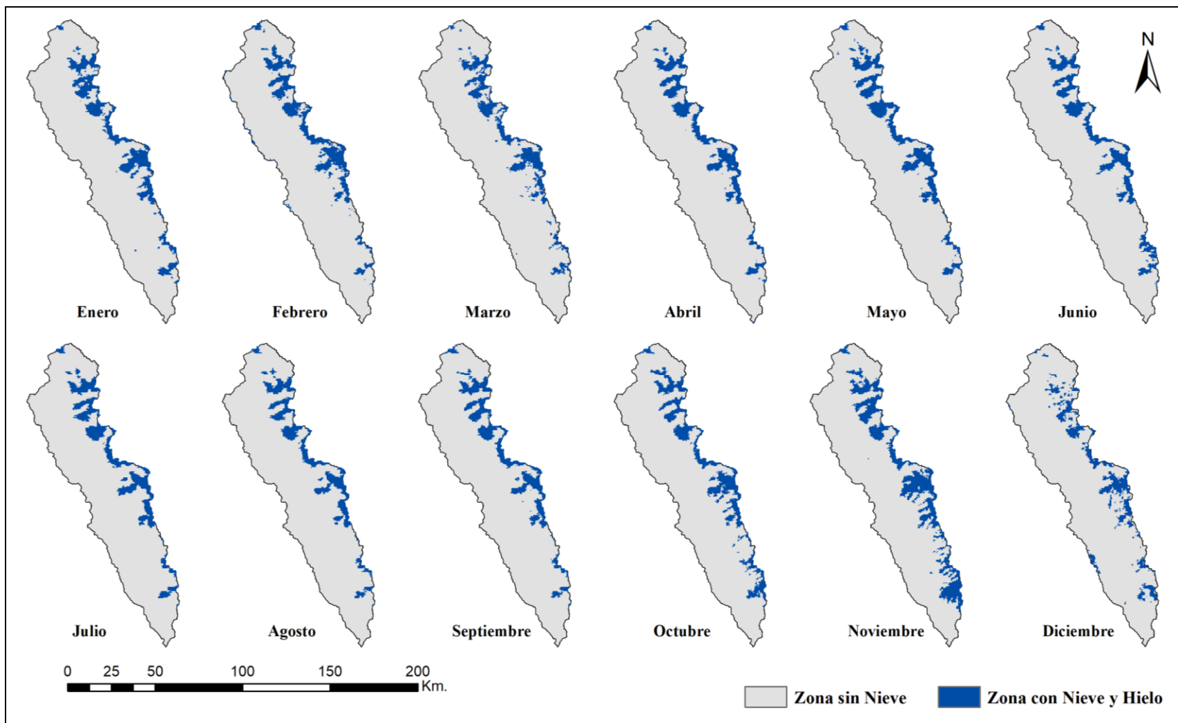
Figura 3.15: Mapas mensuales de cobertura glaciara del año 2010, producto de la imagen de satélite MODIS10A1.
