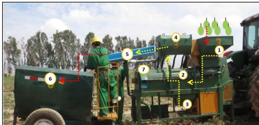
Figura N° 44 Trilladora: 1) Tolva -triturador, 2) Zaranda 3) Bomba de succión, 4) “Finish” (regula cantidad de jugo), 5) Canaleta de salida, 6) Coloso 7) Zona de desfogue (restos de pulpa, cascara)
